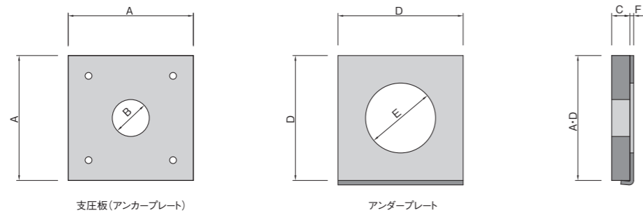
支圧板(アンカープレート)、アンダープレート形状寸法
