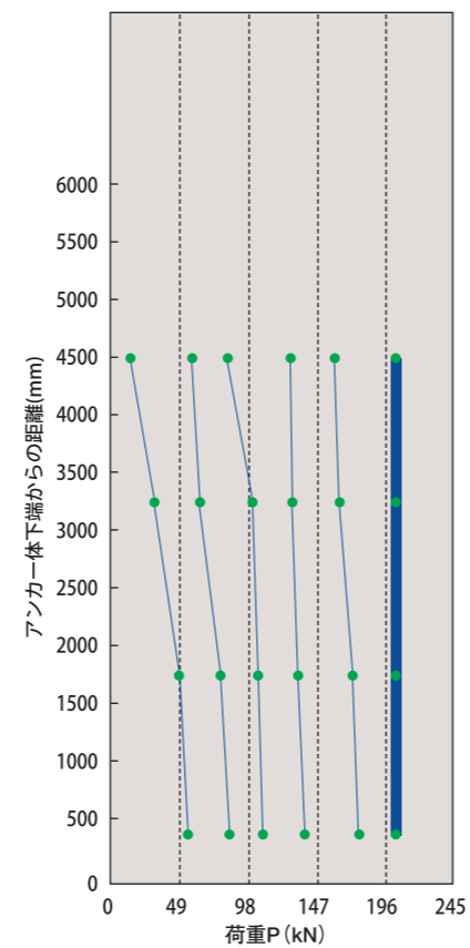
テンドン頭部変位から換算した荷重 全耐力体
