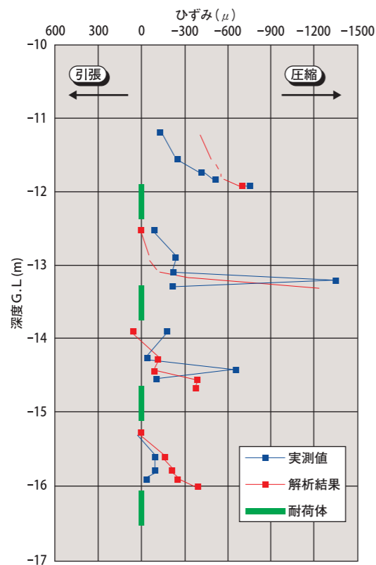
解析定数の変更後の結果(ひずみ分布)
