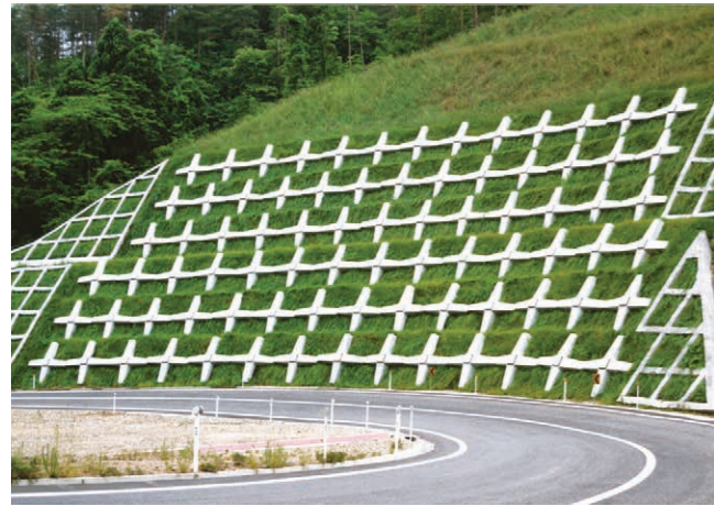
PCフレーム 一般県道特殊改良工事(鳥取県)
