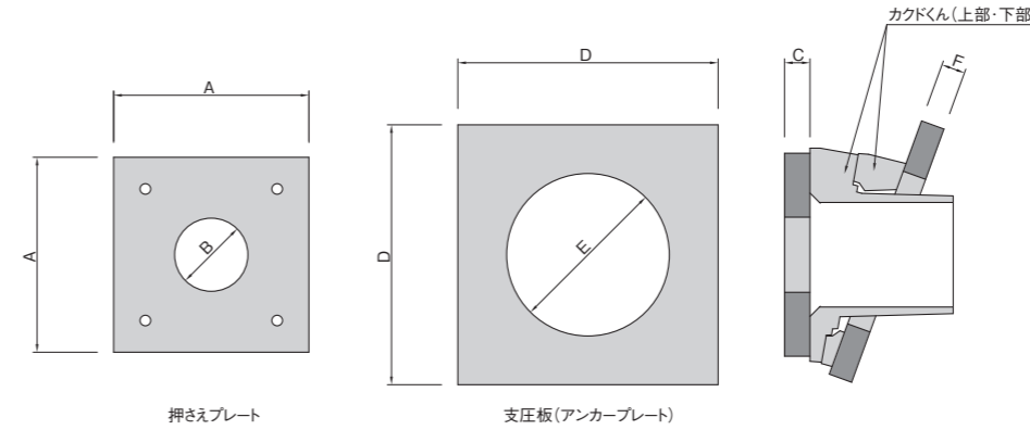
押さえプレート、支圧板(アンカープレート)形状寸法
