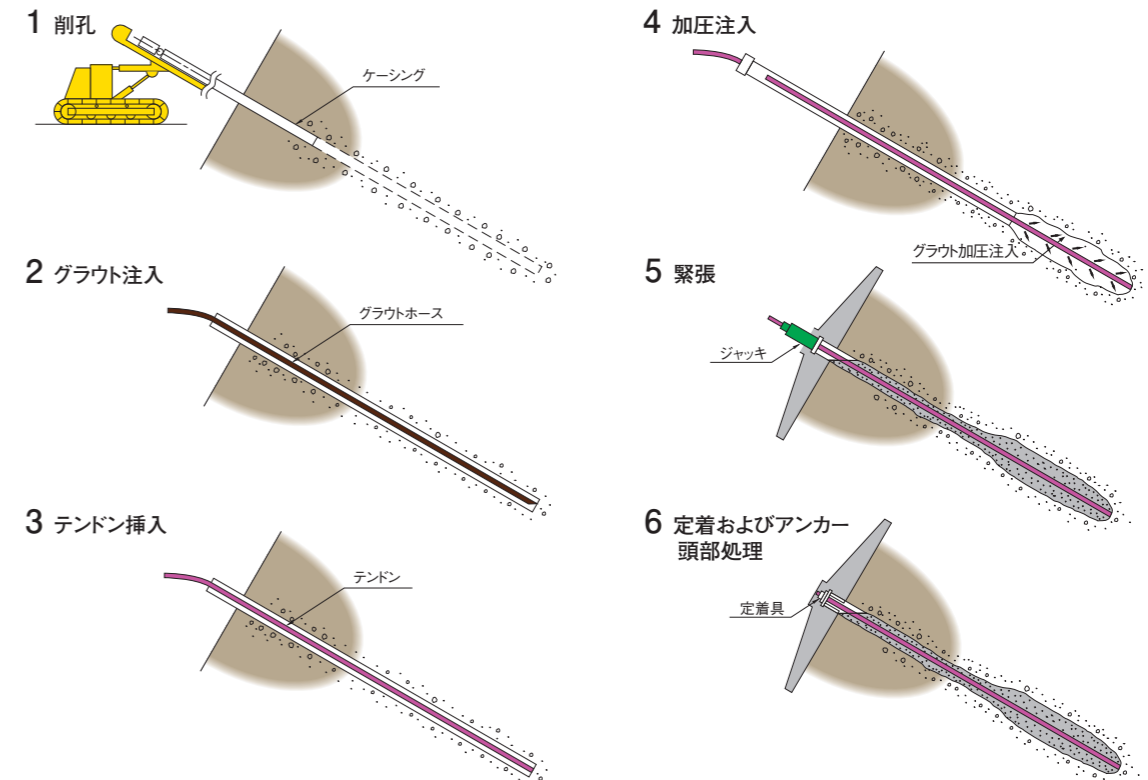
主な作業工程
