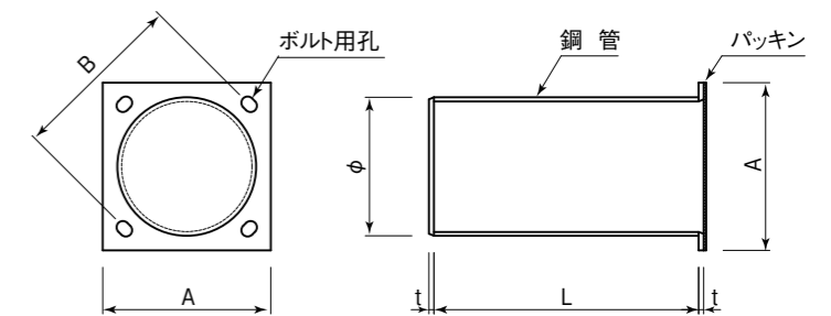
維持管理型鋼製キャップの形状寸法
