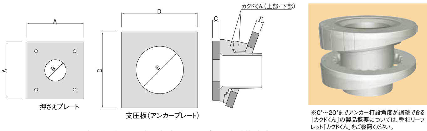
押さえプレート、支圧板(アンカープレート)形状寸法
