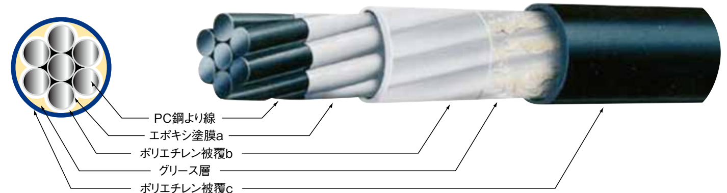
SCアンボンド(SC-U 2 )の塗膜、被覆寸法
