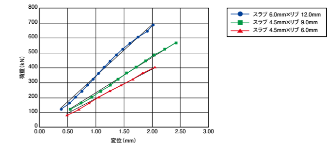
オクトシリーズ載荷試験 荷重-たわみ曲線
